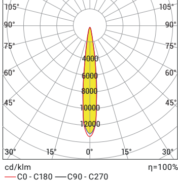
Polar Diyagram - 10°
